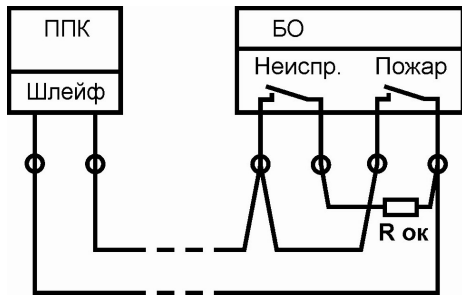
Схема подключения одного извещателя по двухпроводному шлейфу
